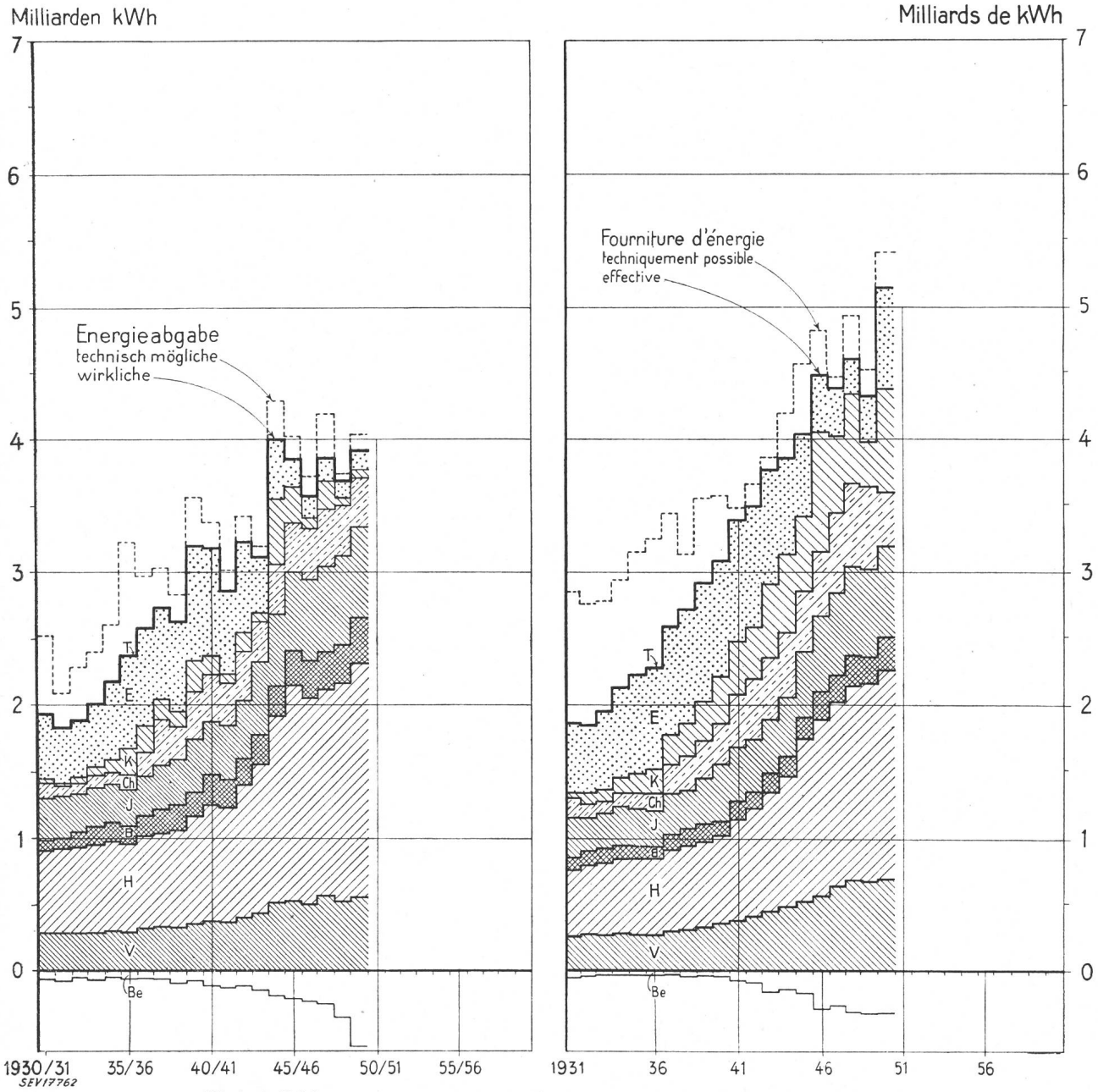
Fig. 2 Sommerhalbjahr (1. April–30. September)
