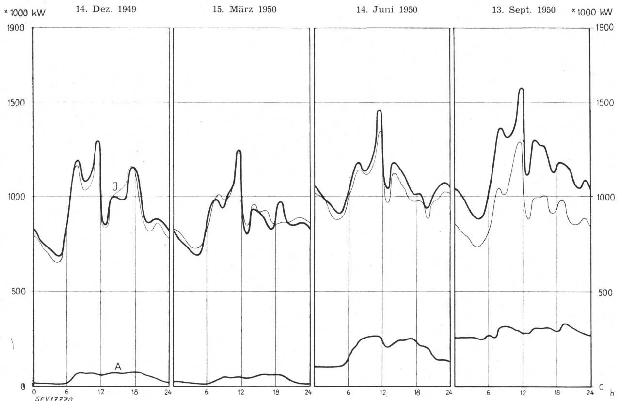
Fig. 7 Verlauf des Inlandverbrauches und der Energieausfuhr an Mittwochen J Inlandverbrauch A Ausfuhr
