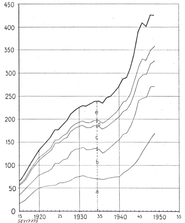
Fig. 12 Jährliche Einnahmen und Ausgaben a Verwaltung, Betrieb und Unterhalt b Abschreibungen und Fondseinlagen c Zinsen und Dividenden d Steuern und Wasserzins e Abgaben an öffentliche Kassen
