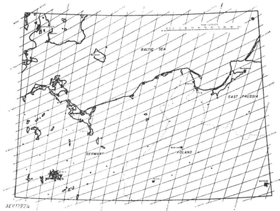
Fig. 10 Loran-Auswertekarte
