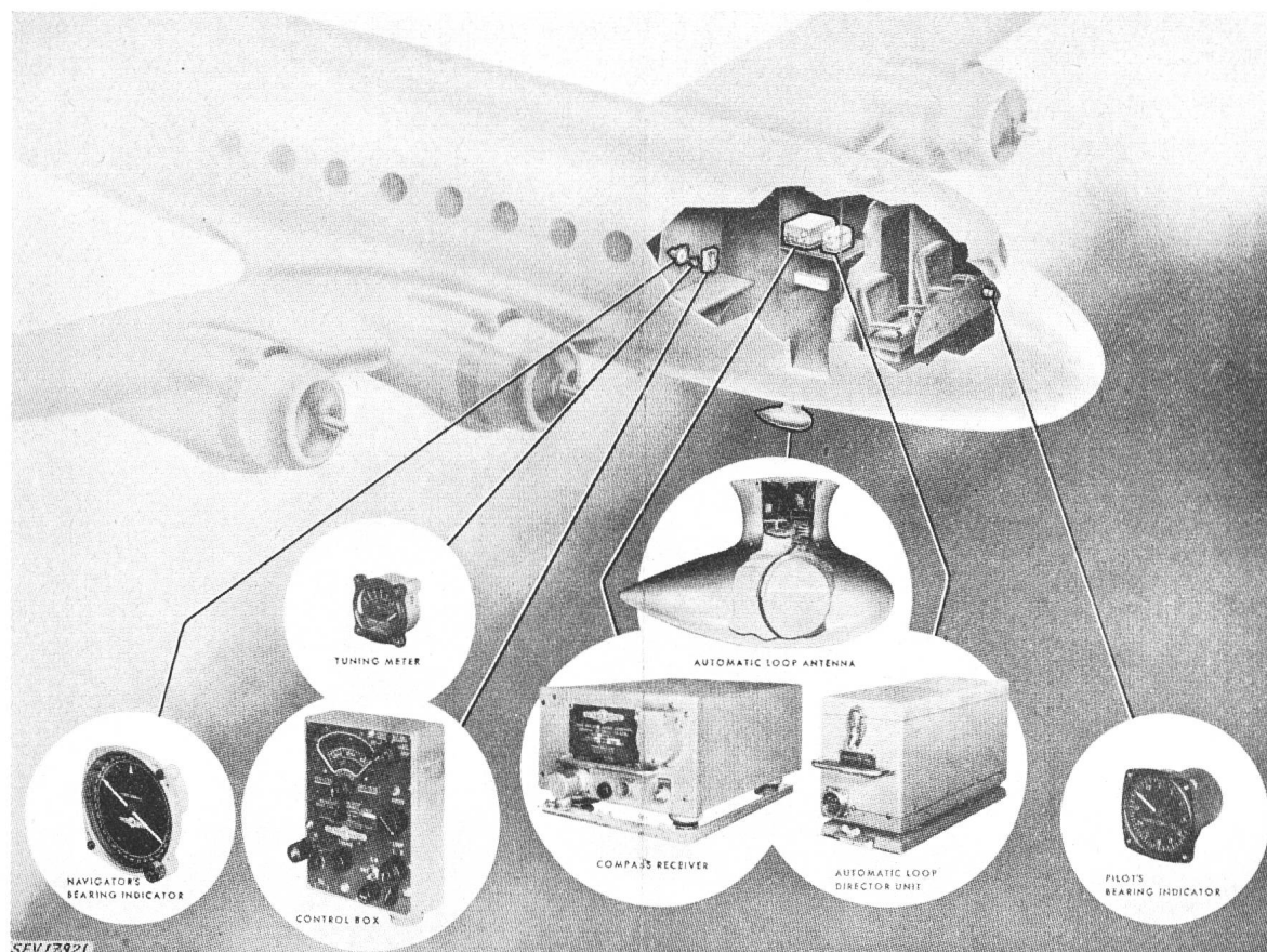
Fig. 7 Automatischer Radiokompass
