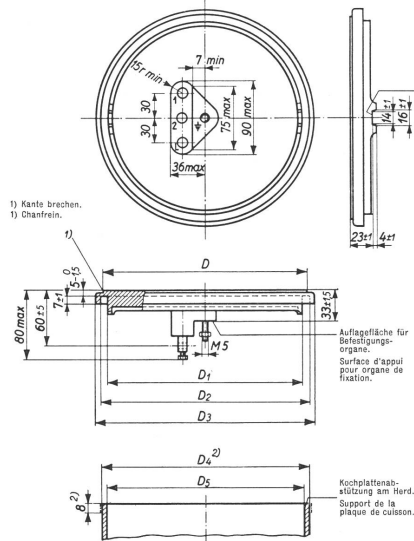
2) Der Durchmesser D 4 darf bis auf das Mass 8 nicht überschritten werden. 2) Jusqu'à la cote 8. Le diamètre D 4 ne doit pas être dépassé.
