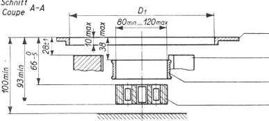
Schnitt A-A
