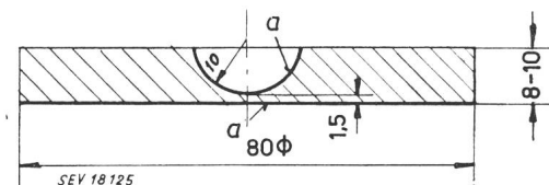
Fig. 4 Porzellan-Prüfkörper zur Bestimmung der Durchschlagfestigkeit a leitender Belag
