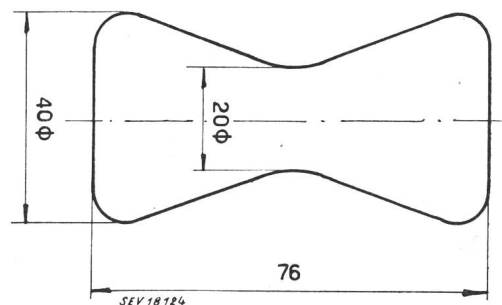
Fig. 3 Porzellan-Prüfkörper zur Bestimmung der Zugfestigkeit
