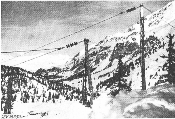
Fig. 9 Lukmanierleitung bei Acquacalda Provisorische Winkelmaße. Jedes Leiterseil ist an einem Baumstamm befestigt
