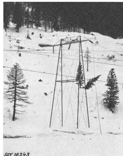
Fig. 2 150-kV-Nufenenleitung
