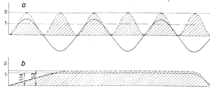
Fig. 14 Vergleich des zeitlichen Verlaufs des Schweißstromes I und der Wärmeleistung I^2R bei gleicher Schweissenergie (Oberwellen vernachlässigt)
