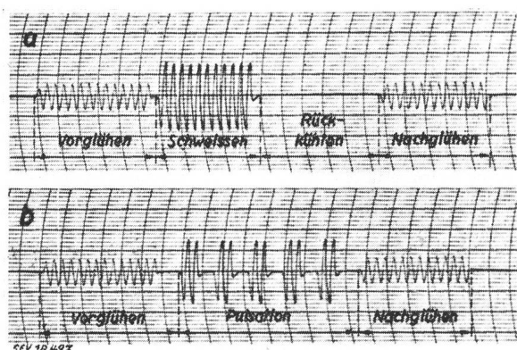
Fig. 11 Oszillogramm des Schweißstromes mit Vor- und Nachwärmstrom a bei Punktschweissung; b bei Pulsationsschweissung
