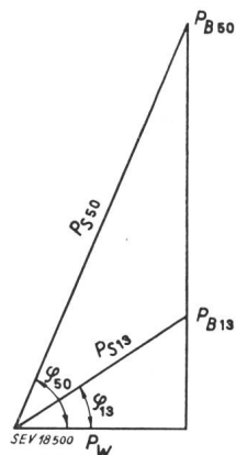
Fig. 13 Leistung und Leistungsfaktor einer 1-Phasenmaschine 50 Hz und einer 3-Phasenmaschine 13 Hz bei gleicher Nutzleistung P_{B50} = 230 kVA; P_{B13} = 65 kVA; P_{S50} = 250 kVA; P_{S13} = 118 kVA; \cos \varphi_{50} = 0,4 ; \cos \varphi_{13} = 0,85 ; P_W = 100 kW
