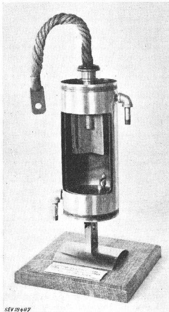
Fig. 1 Ignitron Schatröhre Maximale Schaltleistung 1200 kVA
