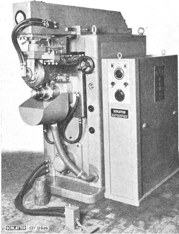
Fig. 8 Nahtschweissmaschine mit elektronischer Synchronsteuerung Schweissleistung 120 kVA
