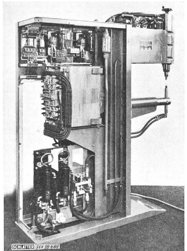
Fig. 2 Punktschweissmaschine für Einzelpunkt- und Repetitionsschweissung mit Ignitronkontakt
