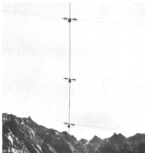
Fig. 6 Queraufhängung
