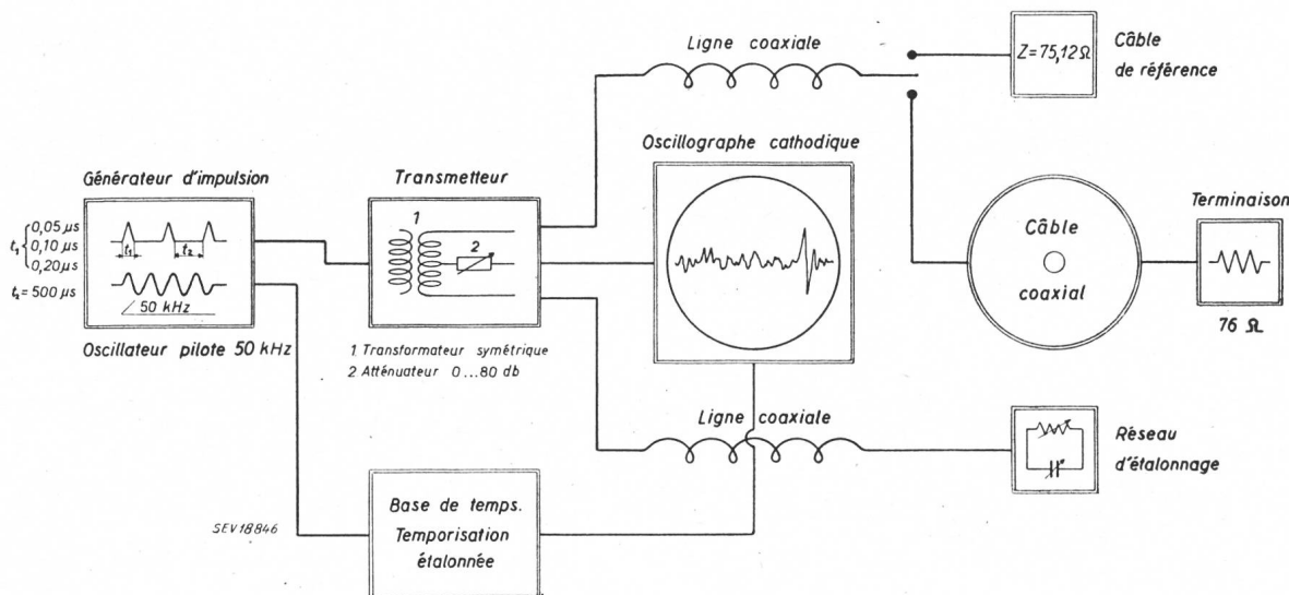
Fig. 3 Schéma de principe d'un appareil de mesure réalisé
