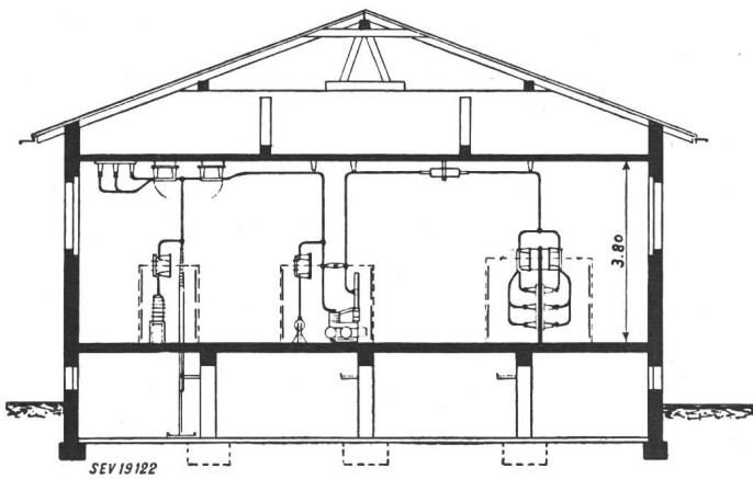
Fig. 5 Querschnitt durch das 16-kV-Schalthaus
