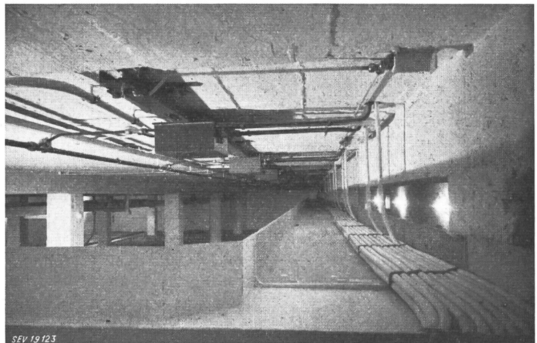
Fig. 6 Anordnungen der Druckluftleitungen und Steuerkabel unter der 16-kV-Schaltanlage
