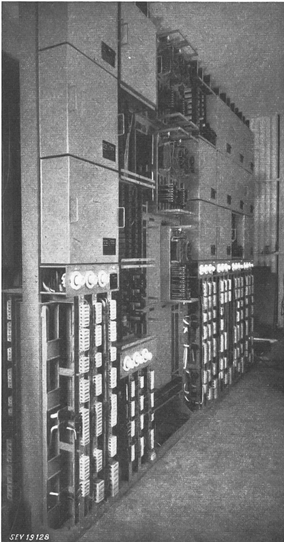
SEV 19128 Fig. 11 Relaisbuchten der Fernsteuerung Verschaltungen teilweise weggenommen
