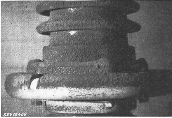
Fig. 9 150-kV-Ableiter mit 5facher normaler Schmutzschicht vollständig durchnässt, mit Leitungswasser von 3000 \Omega\text{cm} ; Schichtdicke ca. 5 mm
