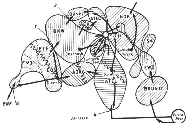
Fig. 6 Schema der Leistungsregulierung bei gegenseitigem Energieaustausch Weitere Bezeichnungen siehe Fig. 1 und 5
