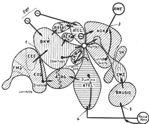
Fig. 5 Schema der Leistungsregulierung 1 Galmiz; 3 Klingnau; 4 Ponte Tresa; 5 Campocolo ⊙ separate Maschinengruppen ~ Auftrennung der Netze RWE Rheinisch-Westfälische Elektrizitätswerke Weitere Bezeichnungen siehe Fig. 1
