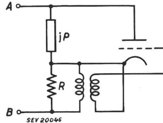
Fig. 4 Tube à réactance Mêmes notations que pour fig. 3
