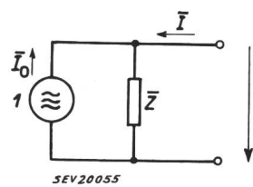
Impédance de sortie d'un amplificateur à deux étages
