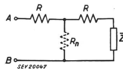
Fig. 5 Transformation d'une impédance Z en une impédance négative \bar{Z}_n par une résistance négative R_n \bar{Z}_n apparaît entre les bornes A et B
