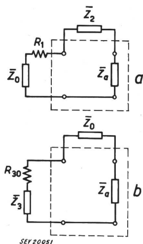
Fig. 9 Impédances négatives connectées à un circuit d'impédance Z_0 a Impédance négative-parallèle b Impédance négative-série Mêmes notations que dans fig. 6 à 8
