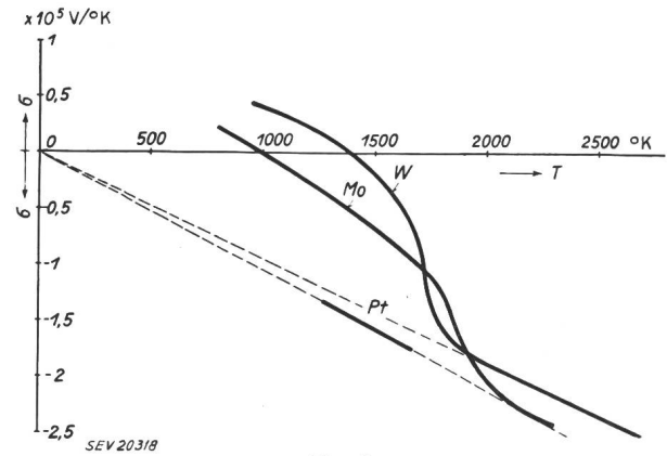
Fig. 7 Thomsonkoeffizient \sigma für W, Mo und Pt in Abhängigkeit von der absoluten Temperatur T
