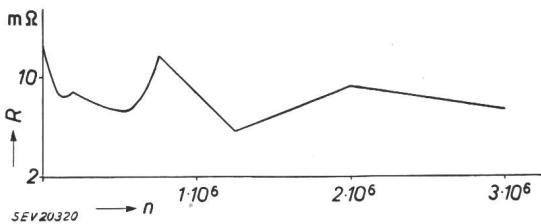
Fig. 9 Kontaktwiderstand von funkenden Silberkontakten R Kontaktwiderstand bei 20 g Druck; n Anzahl Schaltungen
