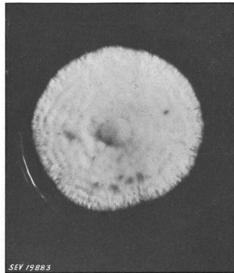
Fig. 1 Merulius lacrimans Wattiges Oberflächenmycel mit typischer Zonenbildung
