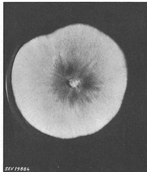
Fig. 2 Coniophora cerebella Dem Nährsubstrat eng aufliegendes Mycel von hellbräunlicher Färbung
