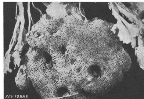
Fig. 6 Fruchtkörper von Poria vaporaria mit charakteristischer Ausbildung der Poren
