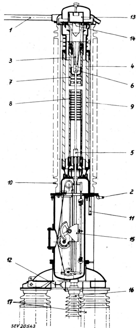
Fig. 2 Schnitt durch eine Schaltkammer des HPF 16 1 Verbindung zwischen den beiden Schaltkammern eines Poles 9 Schaltkammer 2 Anschlussbolzen 10 Porzellanmantel 3 Kontaktträger 11 Ölstandsanzeiger 4 Tulpenkontakt 12 Ölablasshahn 5 Gleitkontakt 13 Ölabscheider 6 Bewegliches Kontaktrohr 14 Sicherheitsmembrane 7 Obere Löschkammer 15 Mechanismus 8 Untere Löschkammer 16 Drehsäule 17 Stützisolatoren
