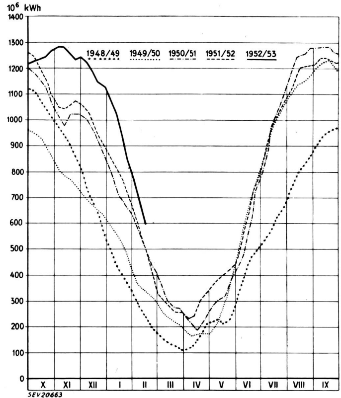
Fig. 10 Energieinhalt der Speicherbecken
