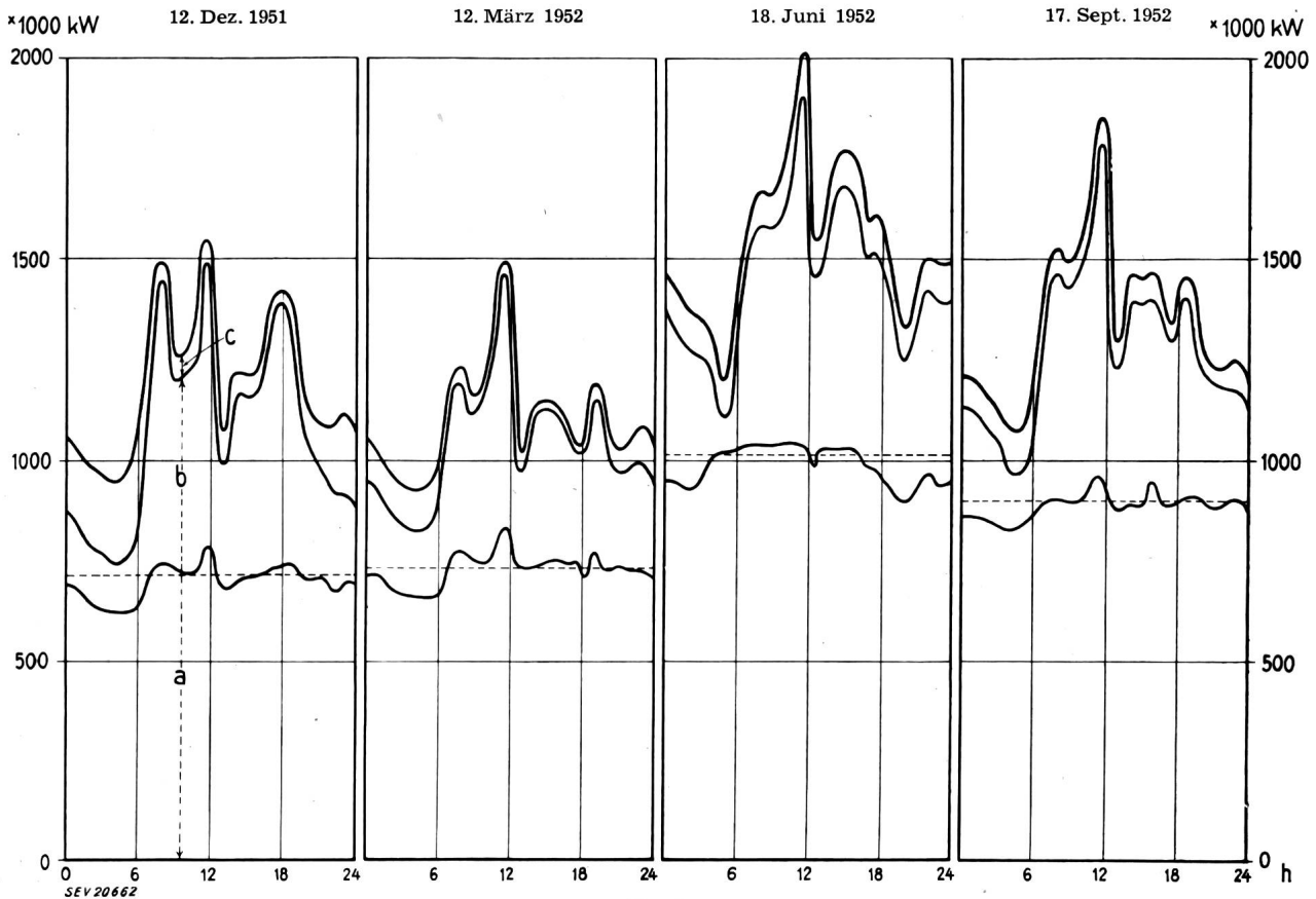
Fig. 9 Verlauf der Energieerzeugung an Mittwochen
