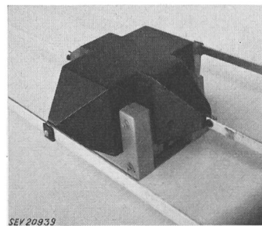
Doppel-Spannungswandler von 20 kV in V-Schaltung ausgeführt als Linientyp
