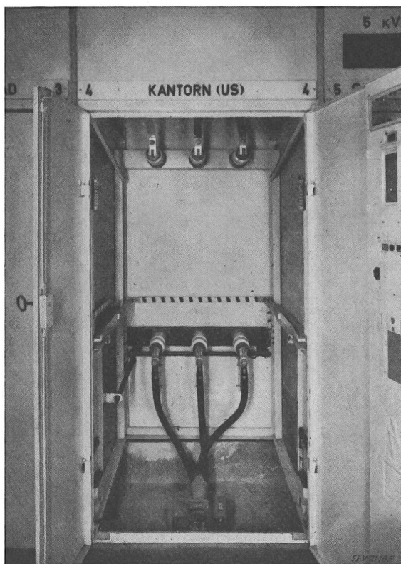
Fig. 5 Schaltfeld mit ausgefahrenem Schaltwagen
