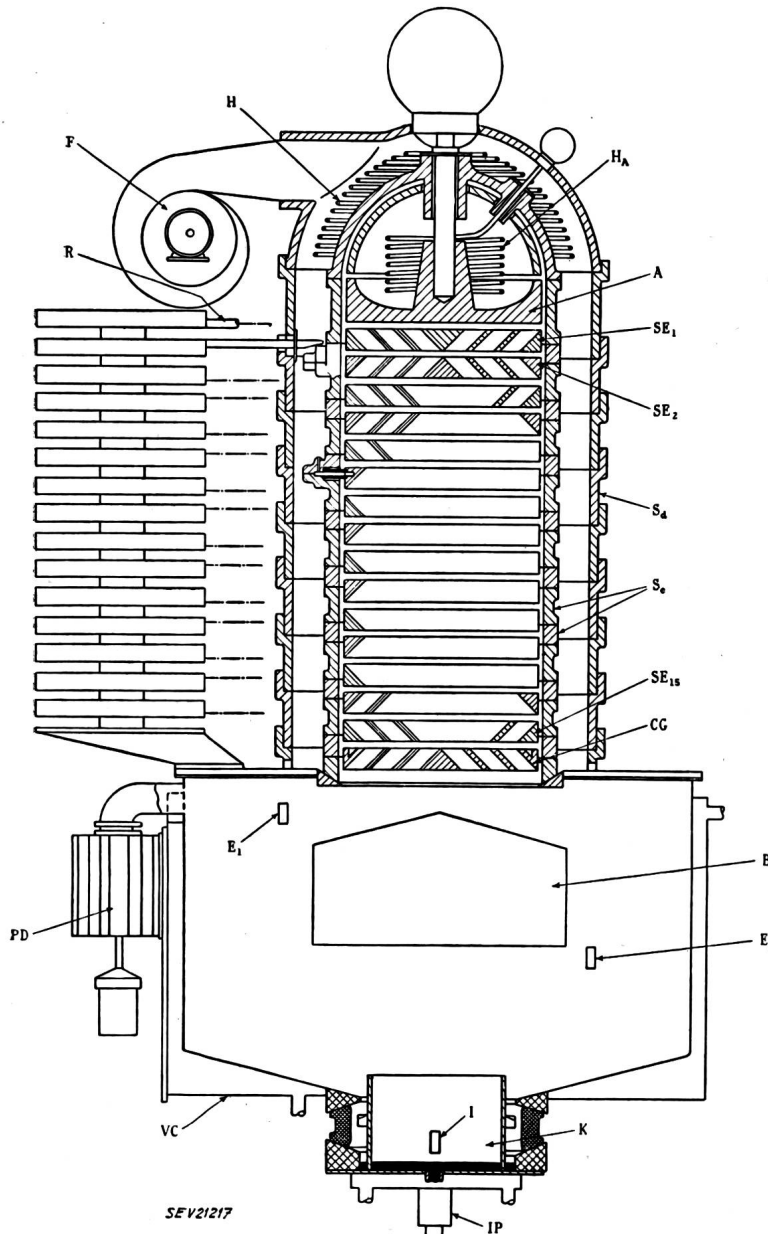
Fig. 1 Quecksilberdampf-Ventil für Gleichrichter- und Wechselrichter-Betrieb
