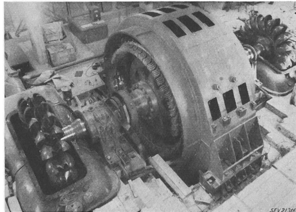
Fig. 1 Maschinensaal Grimsel des Kraftwerkes Oberaar Montagezustand am 13. Januar 1953
