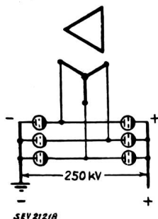
Fig. 2 Dreiphasen-Brückenschaltung mit 6 Gleichrichter-Wechselrichter-Ventilen für Umformen von Wechselstrom in Gleichstrom von 250 kV und umgekehrt
