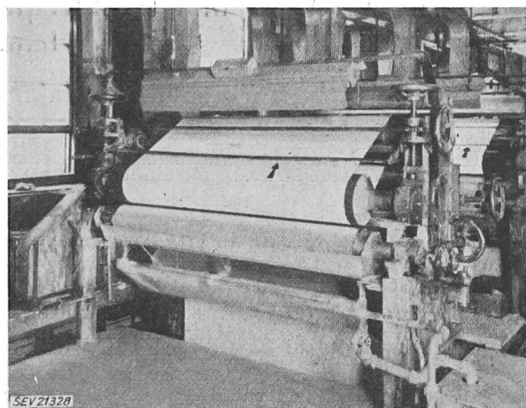
Fig. 2 Elektrostatischer Eliminator auf einer Heliographie-Rotationspresse in einer Druckerei Die Eliminatoren sind durch Pfeile gekennzeichnet
