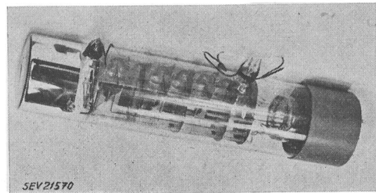
Fig. 10 12stufiger Vervielfacher
