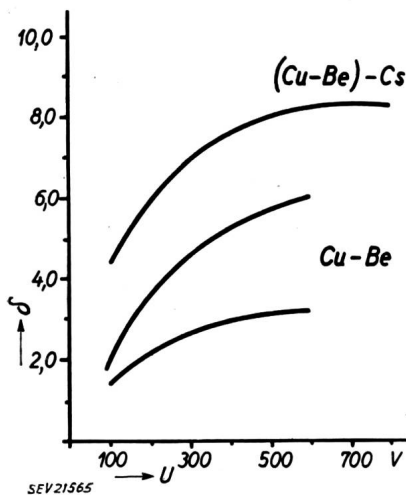
Fig. 5 Ausbeutekurven von Cu-Be-Dynoden δ Verstärkungsfaktor; U Beschleunigungsspannung der primären Elektronen
