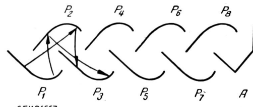
Fig. 7 Schematischer Aufbau des Vervielfachers in Fig. 6 A Anode; P 1 ...8 Dynoden
