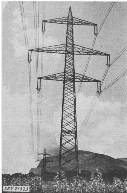
Fig. 1 Tragmast
