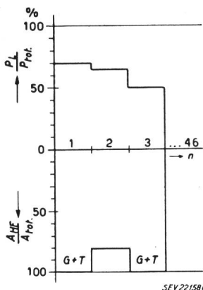
Fig. 3 Gruppe I, Netzpunkte mit Kurzschlussleistungen bis 400 MVA Gesamtzahl der Netzpunkte: n = 46 Zahl der Netzpunkte mit \frac{P_L}{P_{tot}} \geq 50\% : 3 Relative Anteile der lokal erzeugten Kurzschlussleistung \frac{P_L}{P_{tot}} und der Amplitude der Schwingung hoher Eigenfrequenz \frac{AHF}{A_{tot}}
