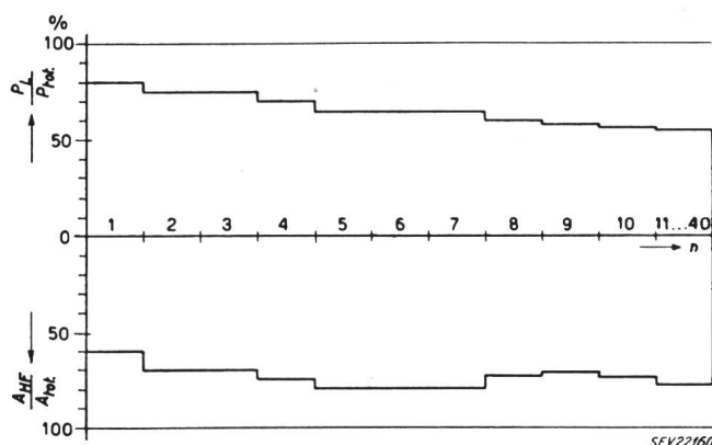
Fig. 5 Gruppe III, Netzpunkte mit Kurzschlussleistungen von 600...1000 MVA Gesamtzahl der Netzpunkte: n = 40 Zahl der Netzpunkte mit \frac{P_L}{P_{tot}} \geq 50\% : 11 Relative Anteile der lokal erzeugten Kurzschlussleistung \frac{P_L}{P_{tot}} und der Amplitude der Schwingung hoher Eigenfrequenz \frac{AHF}{A_{tot}}
