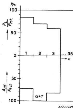
Fig. 4 Gruppe II, Netzpunkte mit Kurzschlussleistungen von 400...600 MVA Gesamtzahl der Netzpunkte: n = 38 Zahl der Netzpunkte mit \frac{P_L}{P_{tot}} \geq 50\% : 3 Relative Anteile der lokal erzeugten Kurzschlussleistung \frac{P_L}{P_{tot}} und der Amplitude der Schwingung hoher Eigenfrequenz \frac{AHF}{A_{tot}}
