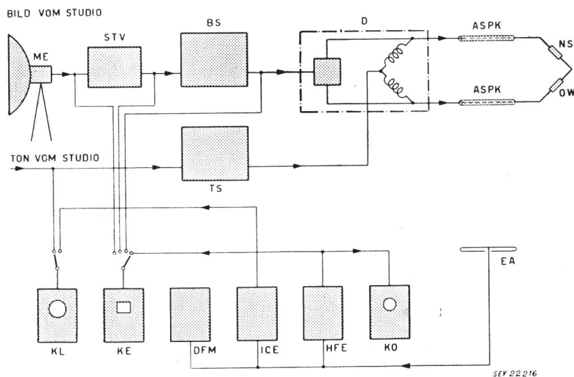
Fig. 4 Blockschema der Sendeanlage auf dem Uetliberg
