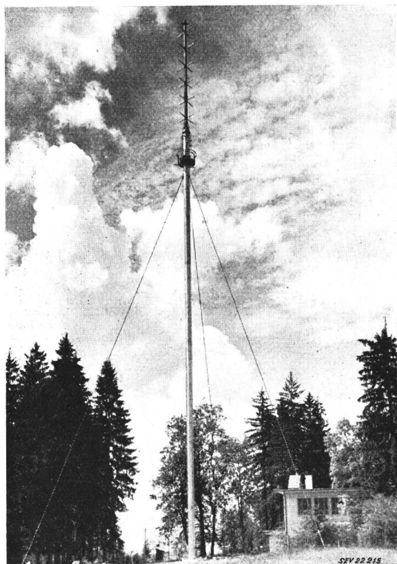
Fig. 3 Fernsehsender Uetliberg
