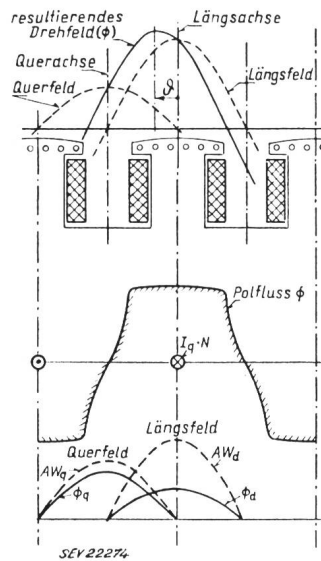
Fig. 3 Feldverteilung der Synchronmaschine \vartheta Polradwinkel; I_q \cdot N Durchflutung in der Querachse; AW_d Ampèrewindungen der Längsachse; AW_q Ampèrewindungen der Querachse; \phi_q Querfluss; \phi_d Längsfluss
