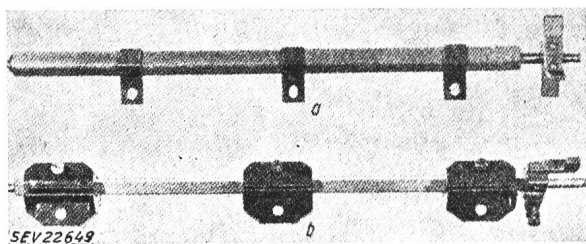
Fig. 4 Auslösewelle
