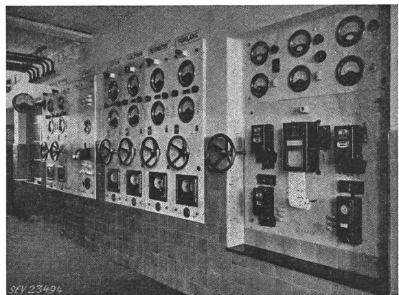
Fig. 2 Alte Schalttafel mit versenkt eingebauten runden Instrumenten
