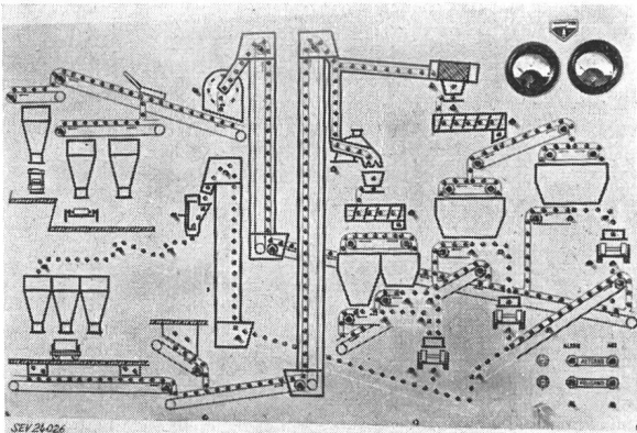
Fig. 5 Leuchtschaltbild einer Sandaufbereitungsanlage
