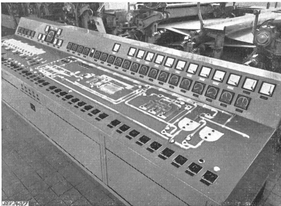
Fig. 6 Kommandopult mit Leuchtschaltbild
