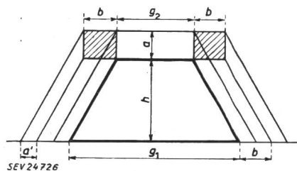
SEV 24726 Fig. 6 Beweis im Fall der Trapeze Differenz der Differenzen \Delta A = 2ab (schraffierte Fläche) Bezeichnungen siehe im Text
