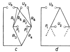
Fig. 7 Schema des Dioden-Multipliziergerätes mit Widerstandswerten Die Werte sind in Ohm angegeben
