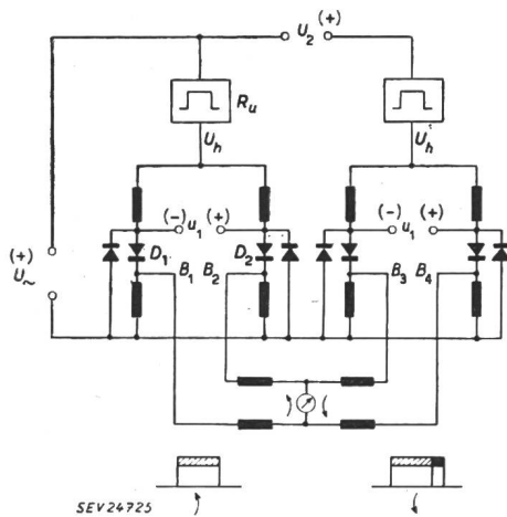
SEV 24725 Fig. 5 Prinzip eines Dioden-Multipliziergerätes
