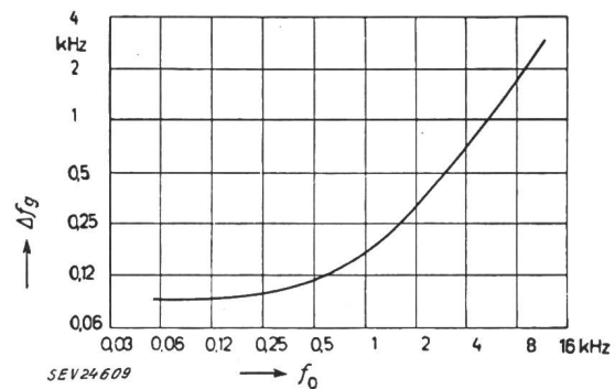
Fig. 3 Breite der Frequenzgruppen
