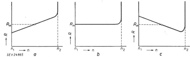
Fig. 1 Schematischer Verlauf des Kontaktwiderstandes R in Funktion der Schaltzahl n
