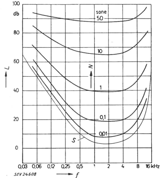
Fig. 2 Mittlere Kurven gleicher Lautheit
