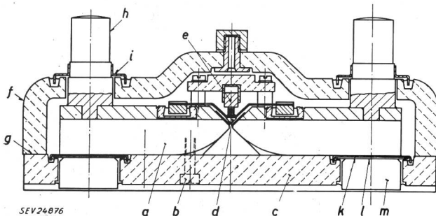
Fig. 6 Gesamtaufbau der Schaltpatrone Maßstab 1 : 1,8
