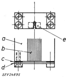
Fig. 5 Frontpartie eines Kontaktpoles a Profilstück; b Polpaket; c Unterlagen 0,03 mm; d Kontaktblech; e eigentliche Kontaktstellen auf dem Kontaktblech
