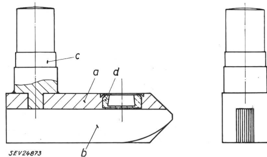
Fig. 3 Kontaktpol
