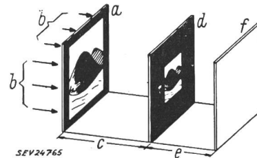
Fig. 2 Anordnung zur Autokorrelation transparenter Vorlagen a transparente Bildvorlage (Diapositiv); b diffuse Lichtquelle; c Abstand der Bildvorlagen von a und d; d eine transparente Bildvorlage von a (Diapositiv) in verkleinertem Massstab; e Abstand der Photoplatte f von der Bildvorlage a
