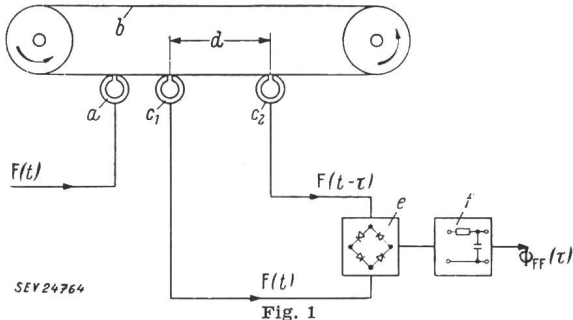
Fig. 1 Analog-Autokorrelator nach dem Tonbandverfahren a Aufsprechkopf; b endloses Magnettonband; c_1, c_2 Abnahmeköpfe; d Abstand zwischen c_1 und c_2 ; e Multiplikator; f integrierendes Glättungsglied Weitere Bezeichnungen siehe im Text
