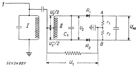
Fig. 1 Frequenz-Diskriminator
