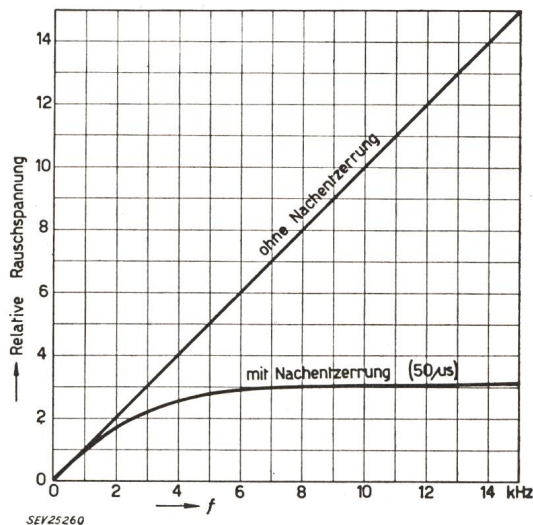
Fig. 8 Rauschspektrum eines FM-Empfängers
