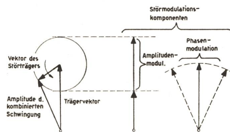
Fig. 3 Störcharakteristik eines diskreten unmodulierten Störträgers 100% Phasenmodulation sei \pm 1 rad, d. h. eine Phasenabweichung, die dasselbe Frequenzband beansprucht wie eine amplitudenmodulierte Übertragung mit identischem Nachrichteninhalt
