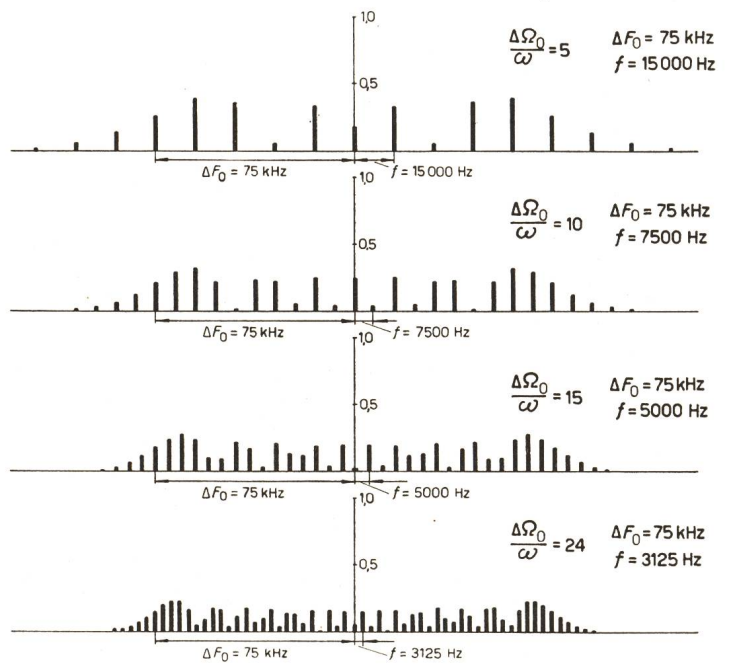
Fig. 1 Seitenbandspektren von FM-Schwingungen links: bei konstanter Modulationsfrequenz f = 5000 Hz und verschiedenen Frequenzhuben \Delta F_0 rechts: bei konstantem Frequenzhub \Delta F_0 = 75 kHz und verschiedenen Modulationsfrequenzen f \Delta \Omega_0 Frequenzhub; \omega Kreisfrequenz der modulierten Schwingung
