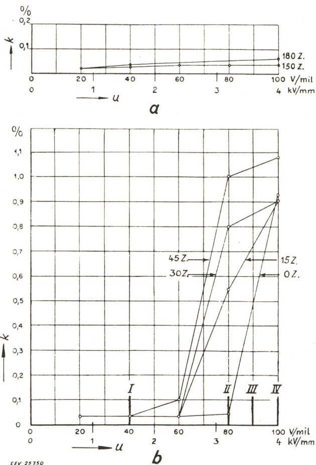
Fig. 1 Messergebnisse von zyklischen Alterungsversuchen an verschiedenen 15-kV-PVC-Kabeln a Alterungsversuch an einem Kabel mit richtig dimensionierter Abschirmung b Alterungsversuch an einem Kabel mit ungeeigneter Dimensionierung der Abschirmung k Verlustfaktor; u Spannungsgradienten (V/mil \equiv V/0,001 Zoll) I Nennspannung; II 2fache Nennspannung; III 2,25fache Nennspannung; IV 2,5fache Nennspannung
