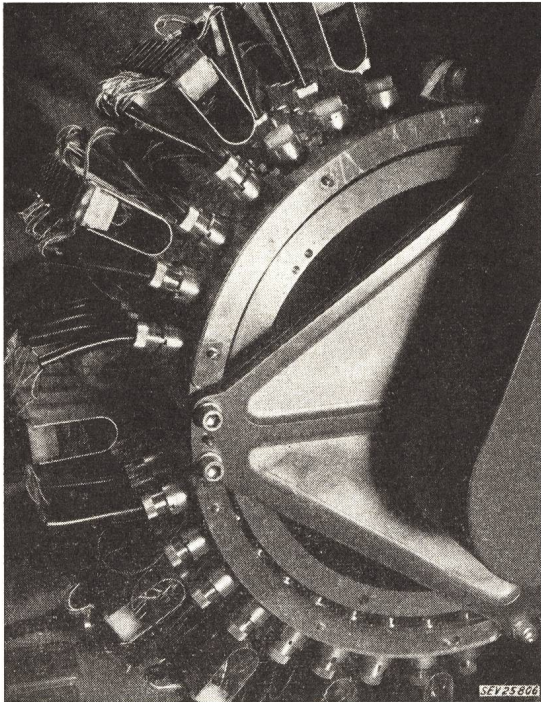
Fig. 6 Teilansicht einer Magnettrommel
