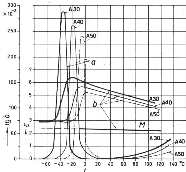
Verlustfaktor (a) und Dielektrizitätskonstante (b) verschiedener Imprägnierungsmittel in Funktion der Temperatur t Temperatur; \text{tg}\delta Verlustfaktor; \epsilon Dielektrizitätskonstante; A30, A40, A50 Typenbezeichnungen für Clophene; M Mineralöl
