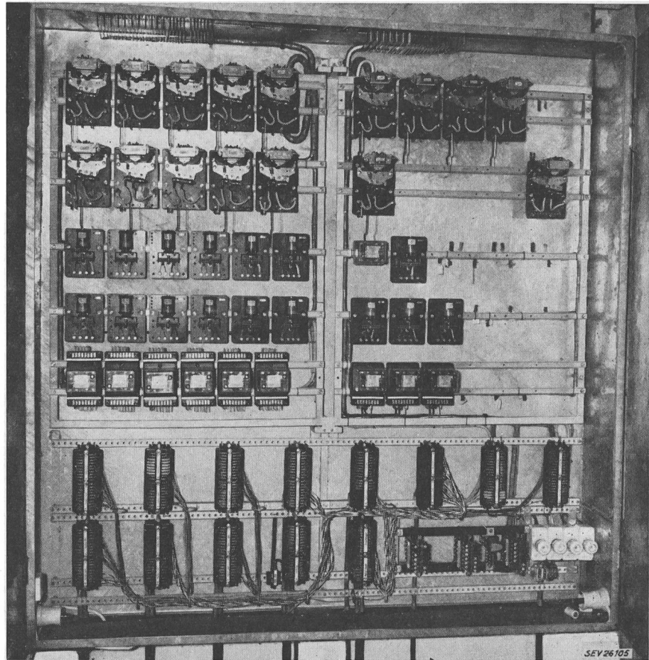
Fig. 5 Steuerrelaiskasten in einer unterirdischen Transformatorstation
