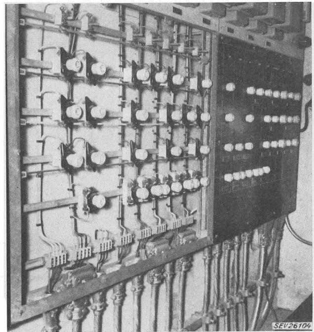
Fig. 4 Sicherungsverteilung in einer unterirdischen Transformatorenstation mit entfernter Abdeckung
