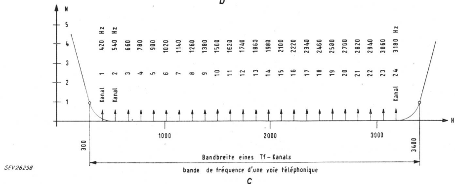
Fig. 10 Spectre de fréquences d'une voie de télégraphie harmonique et schéma de principe de l'émetteur et du récepteur d'une extrémité de voie
