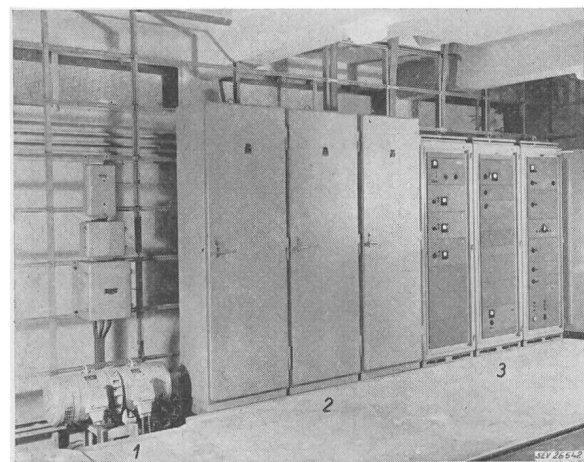
Fig. 12 Fernwirk-Einrichtungen in einem ferngesteuerten Unterwerk Unterwerk Boniswil der Aargauischen Elektrizitätswerke 1 Notstromgruppe; 2 Fernsteuerung (3 Schränke) und Rückmeldung; 3 Trägerfrequenzgerät, geöffnet (1 Schrank), Geräte für Tonfrequenzträger sowie Einzel- und zyklische Fernmessung (2 Schränke)
