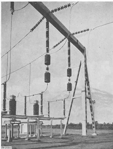
Fig. 11 Anordnung einer Zweiphasenkopplung mit hängenden Kopplungskondensatoren für 220 kV und hängenden Sperren für 1000 A Nennstrom
