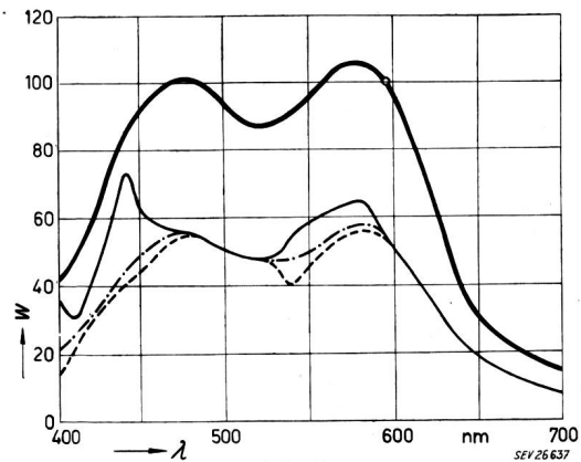
Fig. 3 Darstellung des Spektrums einer «Daylight»-Lampe \lambda Wellenlänge; W relative spektrale Energieverteilung — nicht kompensiert — — — kompensiert - · - · - korrigiert für die korrigierte Kurve ist der Wert des Impulses bei \lambda = 595 nm willkürlich gleich 100 gesetzt; die anderen Impulse sind darauf bezogen worden. Dadurch erhält man die relative spektrale Energieverteilung
