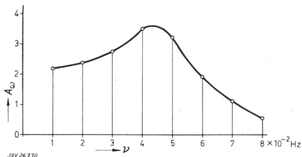
Fig. 4 Spectre de l'agitation de la vitesse A_w amplitude des variations de vitesse; \nu fréquence d'agitation
