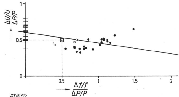
Fig. 9 Mesures à Pierre-de-Plan (Réseau de Lausanne)
