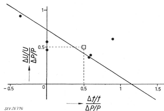
Fig. 10 Mesures à Verbois (Réseau de La Renfile, Genève)
