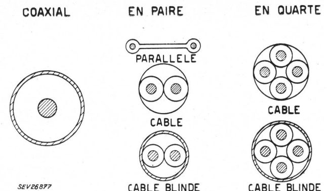
Fig. 1 Kabeltypen
