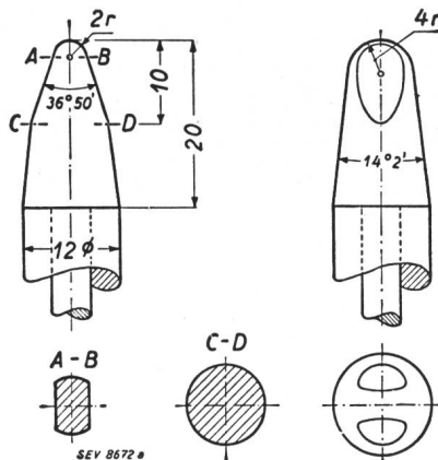
Fig. 6 Tastfinger für die Prüfung der Berührbarkeit unter Spannung stehender Teile
