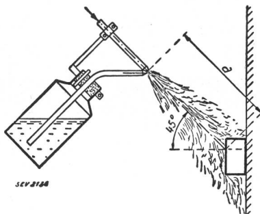
Fig. 8 Zerstäuber für die Beregnung bei der Prüfung auf Feuchtigkeitsbeständigkeit a = 40 \text{ cm}
