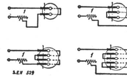
Fig. 9 Schaltungen für die Prüfung auf Stromerwärmung 1 = regulierbarer Widerstand
