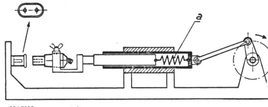
Fig. 2 Apparat für die Prüfung des Verhaltens im Gebrauch a elastisches Zwischenglied
