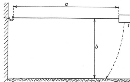
Fig 5 Prüfung der mechanischen Festigkeit von ortsveränderlichen Steckkontakten für industrielle Zwecke a = 225 cm; b = 125 cm 1 = Apparatesteckdose
