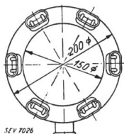
Fig 1 Apparat für die Prüfung der Wärmebeständigkeit a Bohrung für Thermoelement im Schutzkragen und im Kontaktstift
