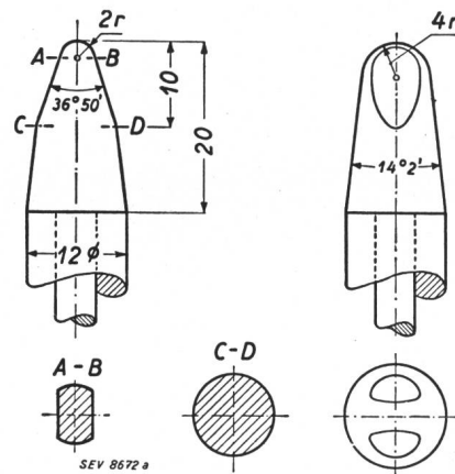
Fig. 10 Tastfinger für die Prüfung der Berührbarkeit unter Spannung stehender Teile Masse in mm
