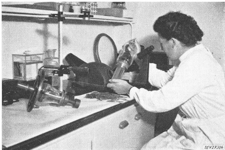
Fig. 4 Spannungsoptische Kontrolle von Glas-Metallverschmelzungen im Polarisoskop
