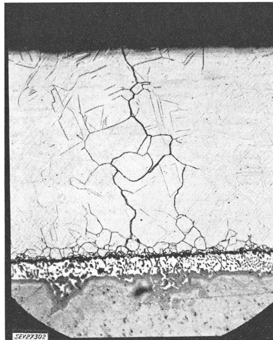
Fig. 2 Lotsprödigkeit bei «Kovar»-Blech Das Lot ist entlang den Korngrenzen ins Gefüge eingedrungen Vergrößerung 150fach
