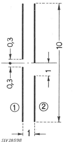
Fig. 15 Malgré l'asymétrie, il n'existe pratiquement pas de composante axiale de la force entre l'ensemble des conducteurs (1) et l'ensemble des conducteurs (2)
