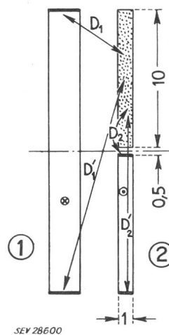
Fig. 16 Considération des distances moyennes géométriques D entre la moitié supérieure de la section (2) et les segments de droite indiqués Pour les désignations, voir les figures précédentes
