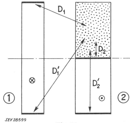
Fig. 16 Considération des distances moyennes géométriques D entre la moitié supérieure de la section (2) et les segments de droite indiqués Pour les désignations, voir les figures précédentes
