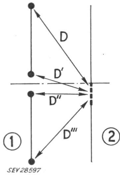
Fig. 14 Distances moyennes géométriques D , D' , D'' et D''' entre les extrêmes des segments qui constituent l'ensemble (1) et la lacune de l'ensemble (2)
