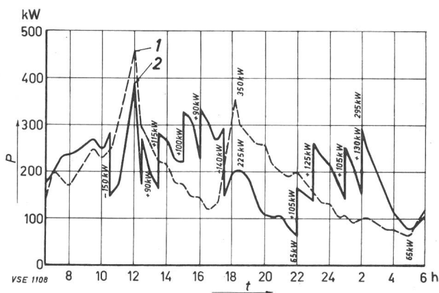
Mit einer Netzkommandoanlage erzielte Verbesserung der Belastungskurve in einem ländlichen und halbstädtischen Niederspannungsverteilnetz
