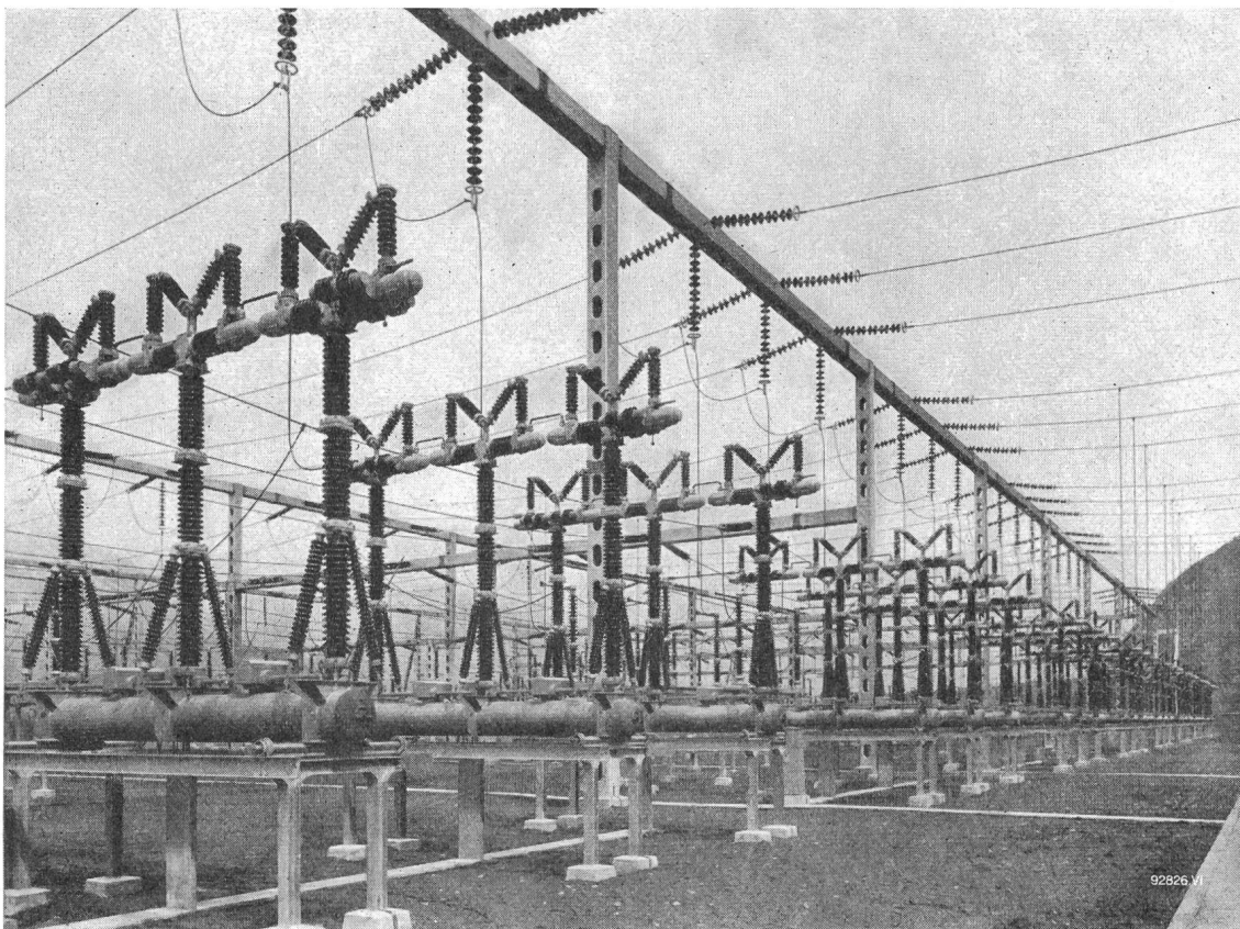
220-kV-Druckluftschneckschalter in der Freiluftanlage des Kraftwerkes Riddes der Forces Motrices de Mauvoisin S.A. Sitten, Wallis
