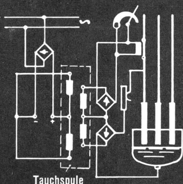
Tauchspule
