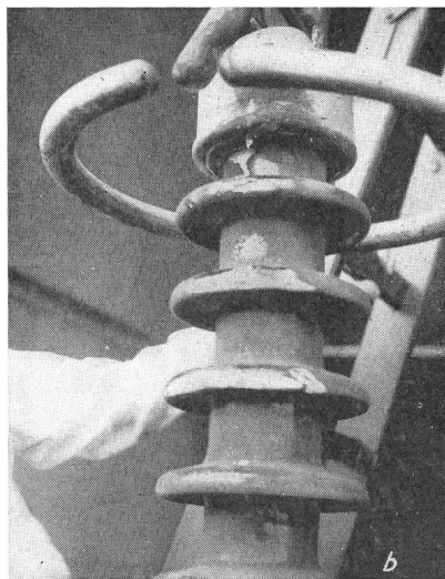
Fig. 5 Zerstörungen an Isolatoren nach einem Lichtbogenüberschlag
