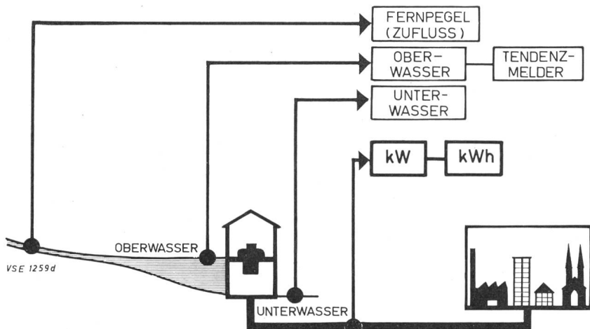
Fig. 2 Vereinfachtes Überwachungsschema für ein Laufkraftwerk
